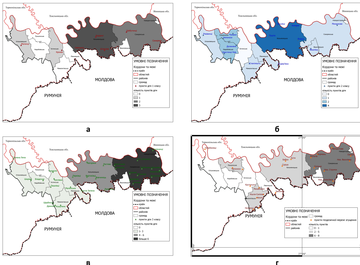
Рис. 2. Просторовий розподіл пунктів ДГМ в розрізі територіальних громад території Дністровського району Чернівецької області
