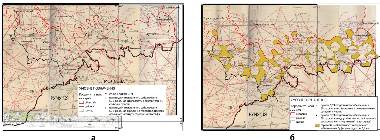
Рис. 4. Територіальний розподіл пунктів ДГМ геодезичного забезпечення 1954–61 років території Дністровського району (а) з векторизованими об'єктами ділянок невідповідності середньої щільності пунктів ДГМ (б)
