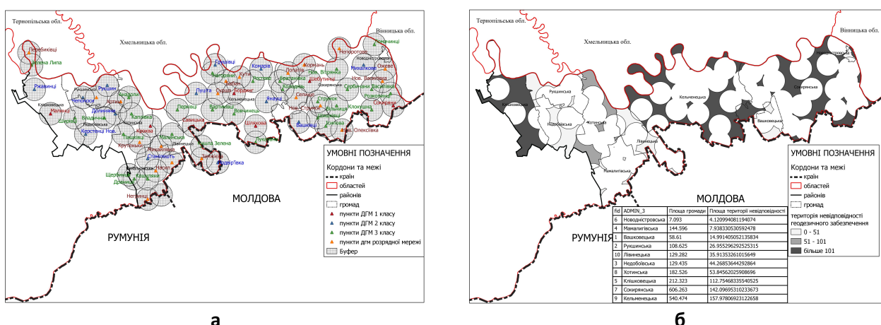
Рис. 3. Картошкама можливості складання карт масштабу 1 : 10 000 (а) для території Дністровського району з векторизованими об'єктами ділянок невідповідності середньої щільності пунктів ДГМ (б)
