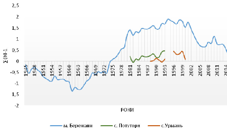
Рис. 5. Різнцева інтегральна крива модульних коефіцієнтів середньої річної кількості опадів (1945–2015 рр.)
