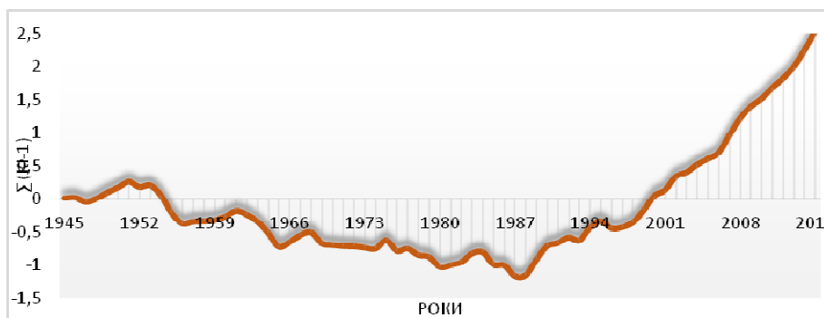
Рис. 2. Різницева інтегральна крива модульних коефіцієнтів показників середньої річної температури повітря (1945–2015 рр.)
