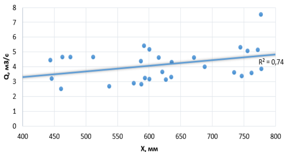
Рис. 6. Графік залежності стоку річки Золота Липа від атмосферних опадів за досліджуваний період
