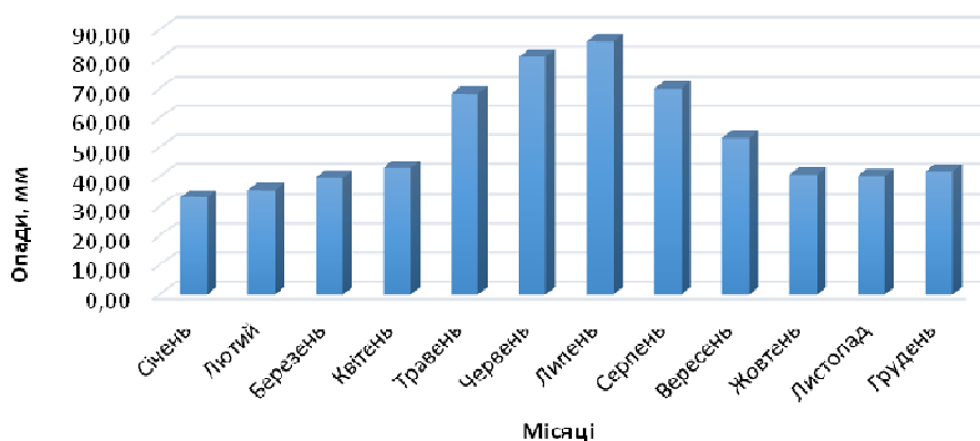
Рис. 3. Середня місячна кількість атмосферних опадів у Бережанському районі протягом 1945–2015 років
